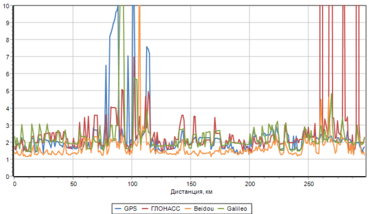
Рисунок 8 Участок 2. Геометрический фактор PDOP (значения выше 10 не показаны)
