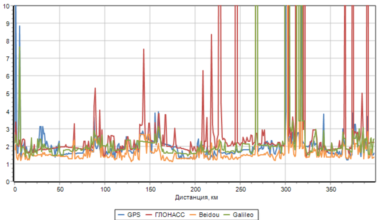
Рисунок 10 Участок 3. Геометрический фактор PDOP (значения выше 10 не показаны)
