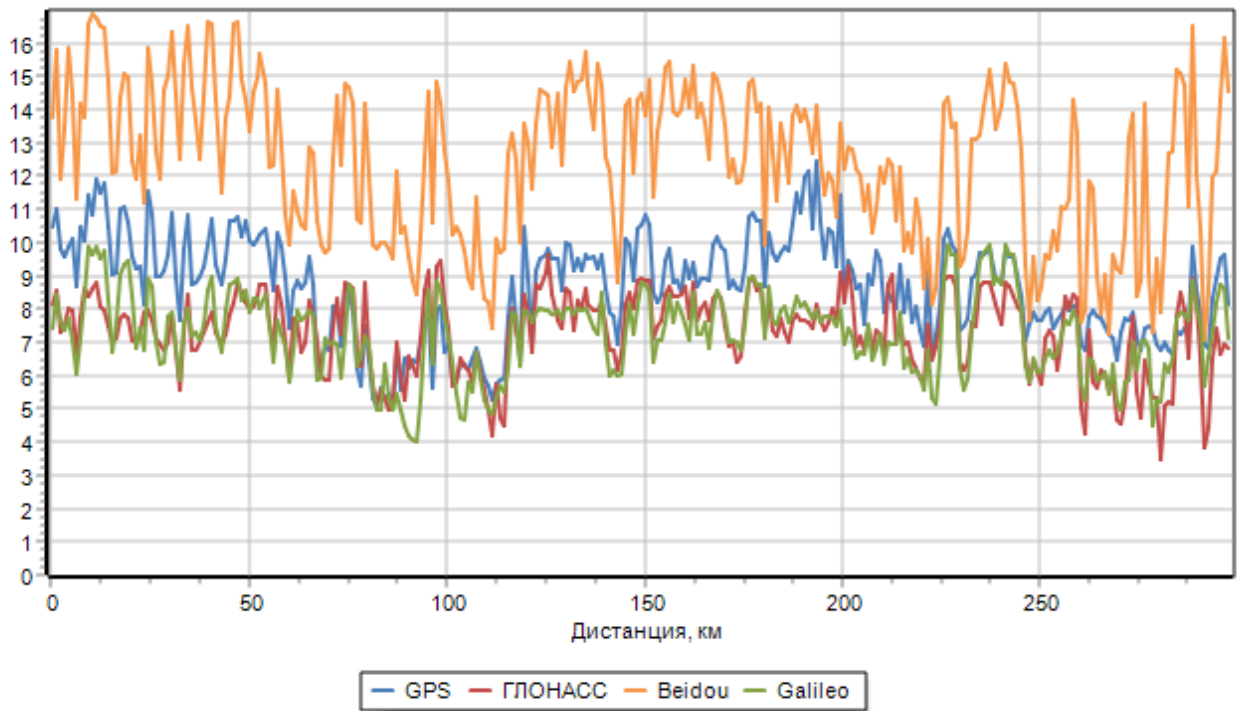
Рисунок 7 Участок 2. Количество видимых НКА
