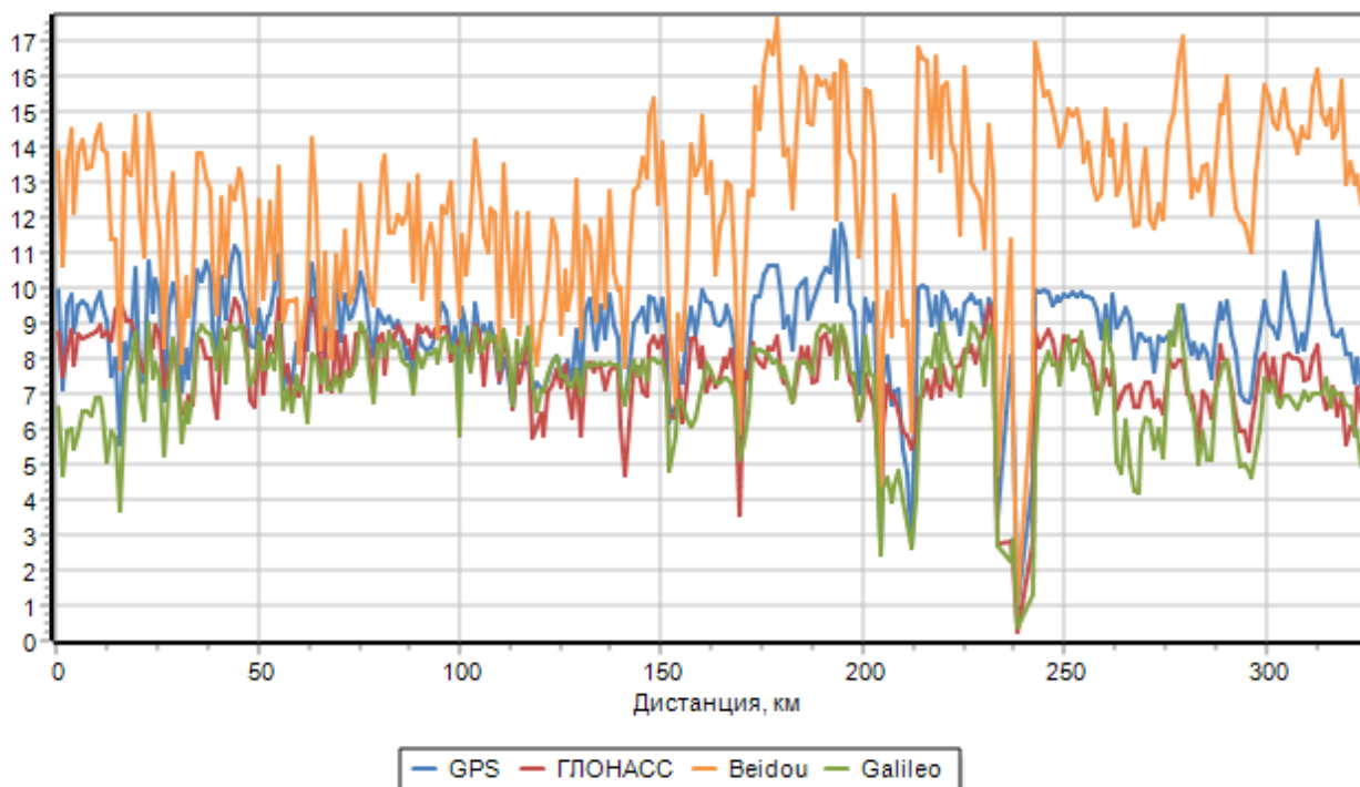
Рисунок 5 Участок 1. Количество видимых НКА
