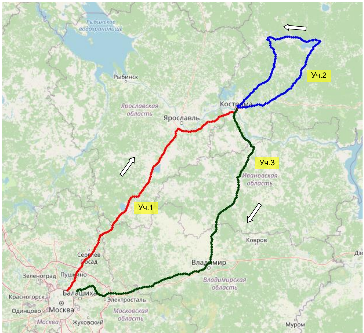
Рисунок 1 Маршрут испытаний
