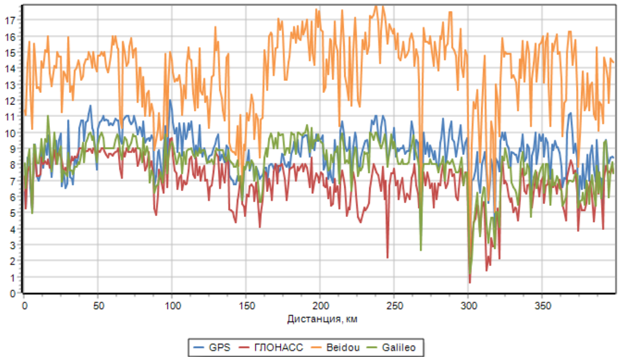
Рисунок 9 Участок 3. Количество видимых НКА
