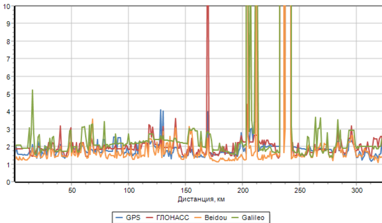
Рисунок 6 Участок 1. Геометрический фактор PDOP (значения выше 10 не показаны)
